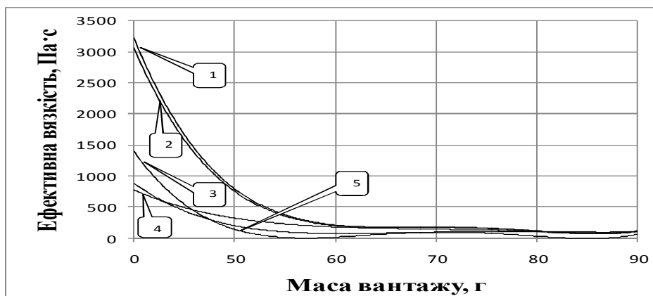
Рис. 2. Ефективна в'язкість ковбасних виробів
