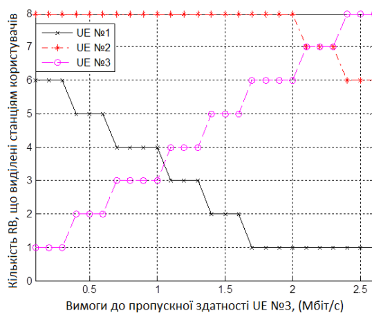
Рис. 7. Залежність кількості ресурсних блоків, що виділяються станціям користувачів від зміни необхідного значення пропускної здатності третьої UE
