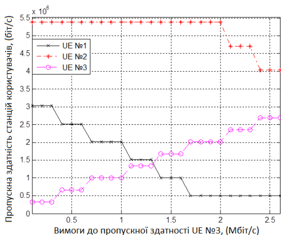
Рис. 6. Залежність пропускних здатностей, що виділяються станціям користувачів від зміни необхідної пропускної здатності третьої UE
