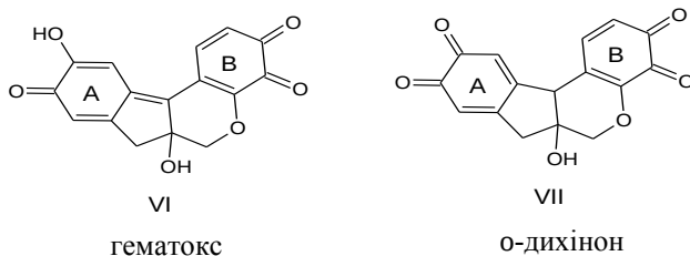
У лужному середовищі при надлишку кисню відбувається окиснення гематоксиліну, яке приводить до утворення гематоксу (VI), о-дихінону (VII) (рис. 2), а також до процесів гідроксилювання, димерізації і окисного розриву кільця.
